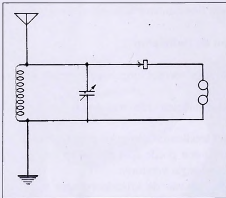
Principe schema van een kristalontvanger of Galènepost
