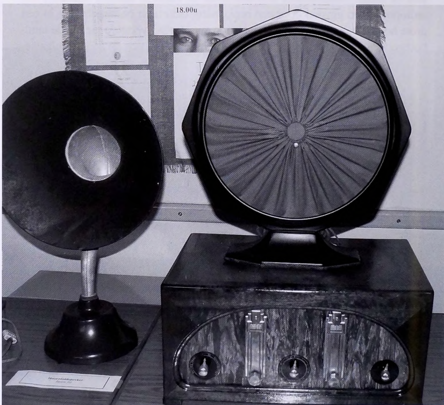
Batterijpost met metalen luidspreker "Sonocorde", beiden van 1925. Links een hoornluidspreker daterend van de jaren 20. (verzameling Luc Van Nevel)
