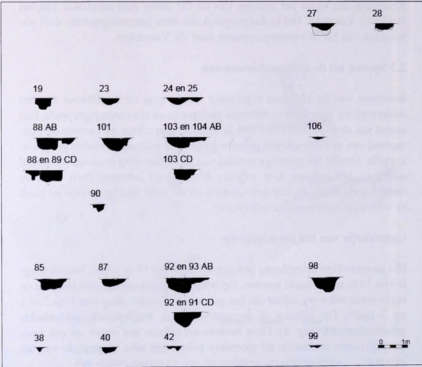
Fig. 5 Overzicht van de coupes op de paalsporen.
